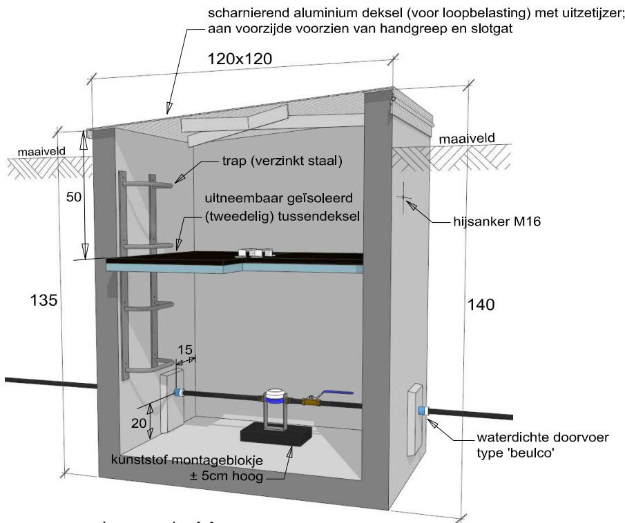
doorsnede AA
