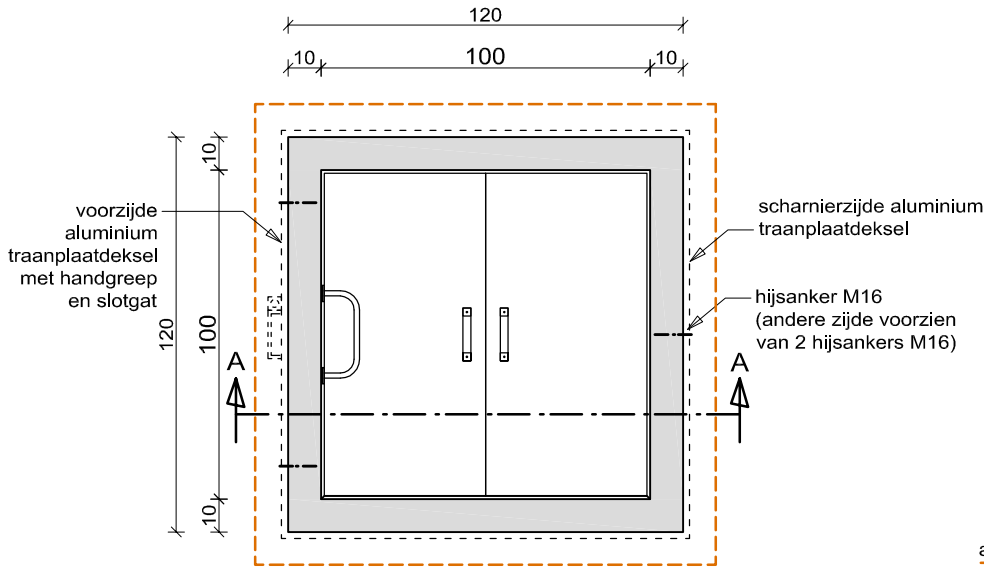
bovenaanzicht (excl. aluminium deksel)
