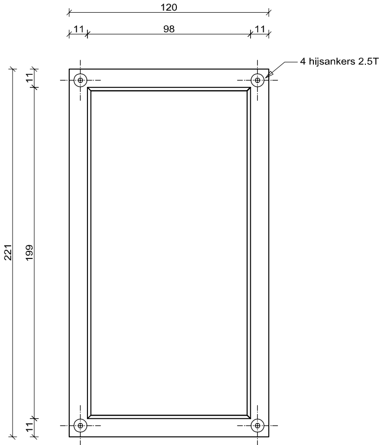
bovenaanzicht
