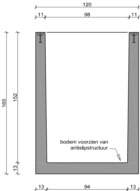
dwarsdoorsnede
