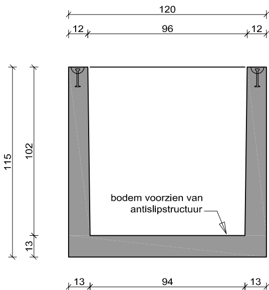
dwarsdoorsnede
