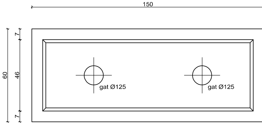
bovenaanzicht
