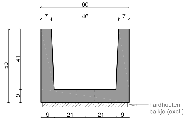
dwarsdoorsnede
