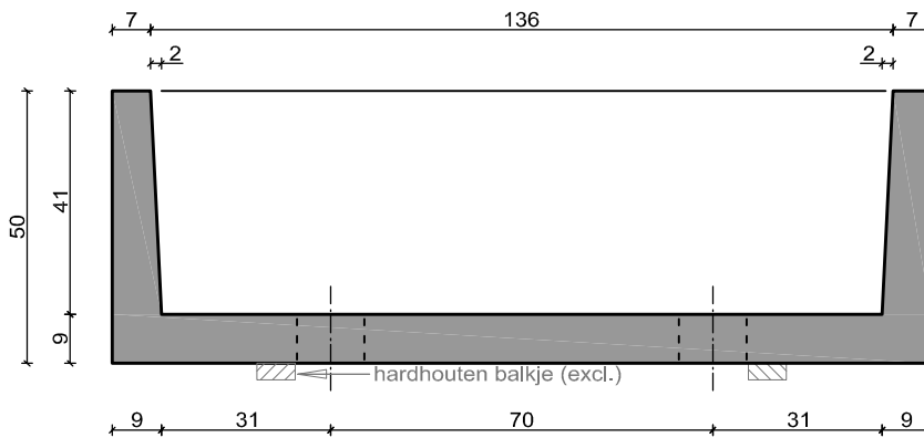
lengtedoorsnede
