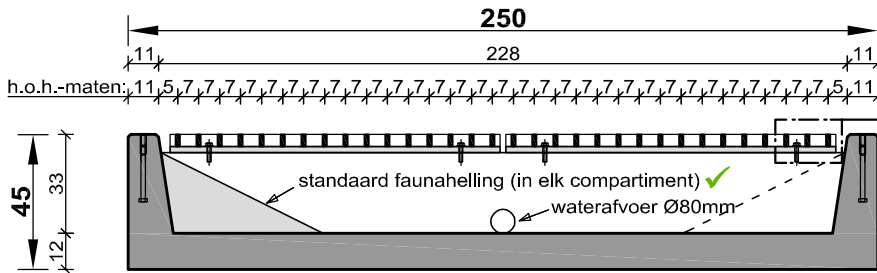
dwarsdoorsnede AA
