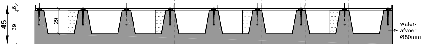
lengtedoorsnede BB
