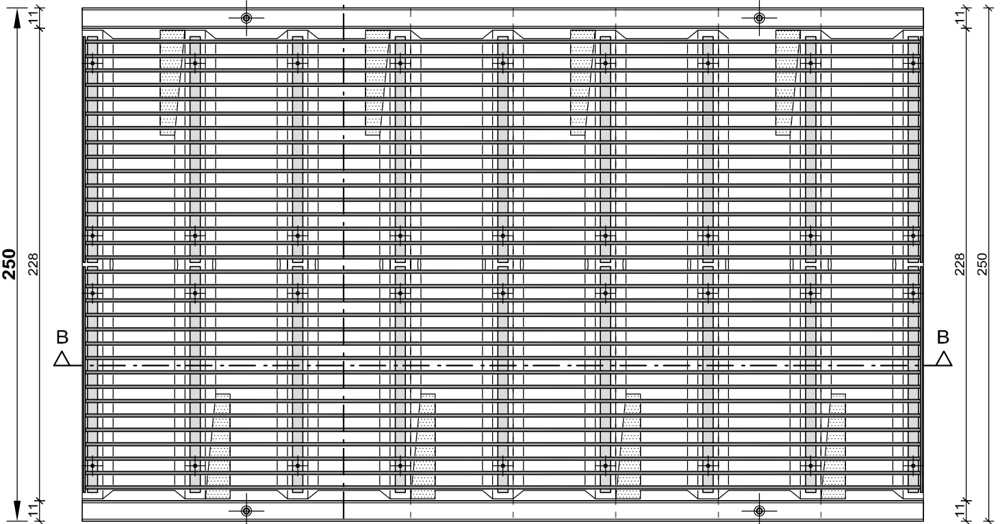
bovenaanzicht
